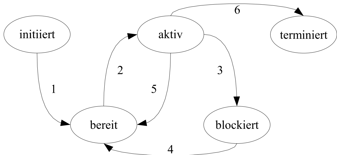
Abbildung 6.2: Prozesszustände
