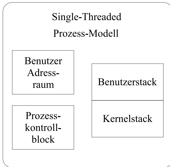
Abbildung 6.3: Single-Thread-Prozess-Modell
