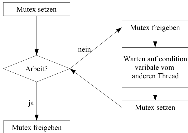
Abbildung 6.5: Condition Variable
